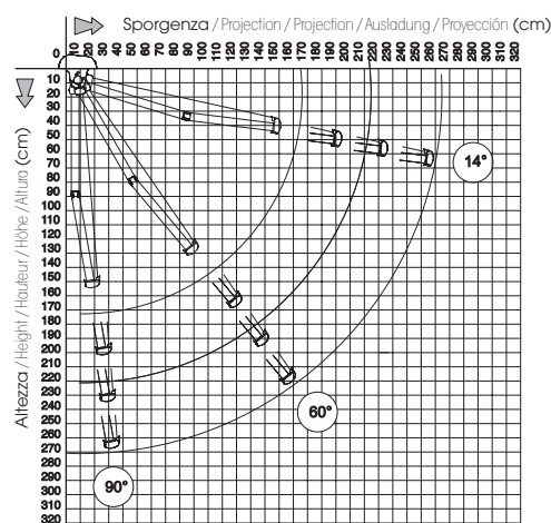
Montaggio a soffitto / Ceiling installation
